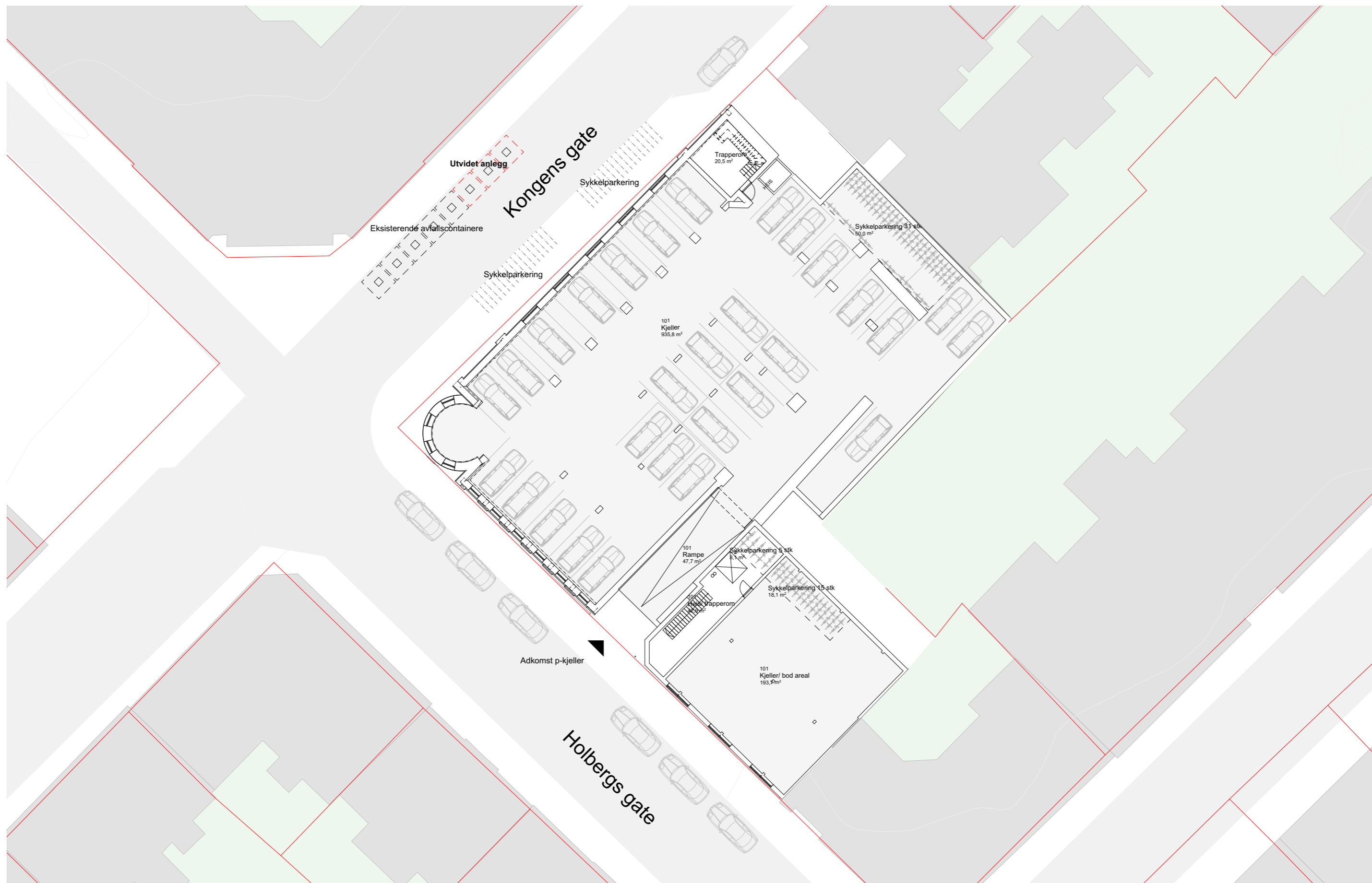
1:300 Parkeringsplan
